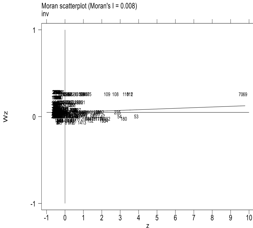
شکل ۱. نمودار پراکنش موران ماخذ: یافته‌های پژوهش
