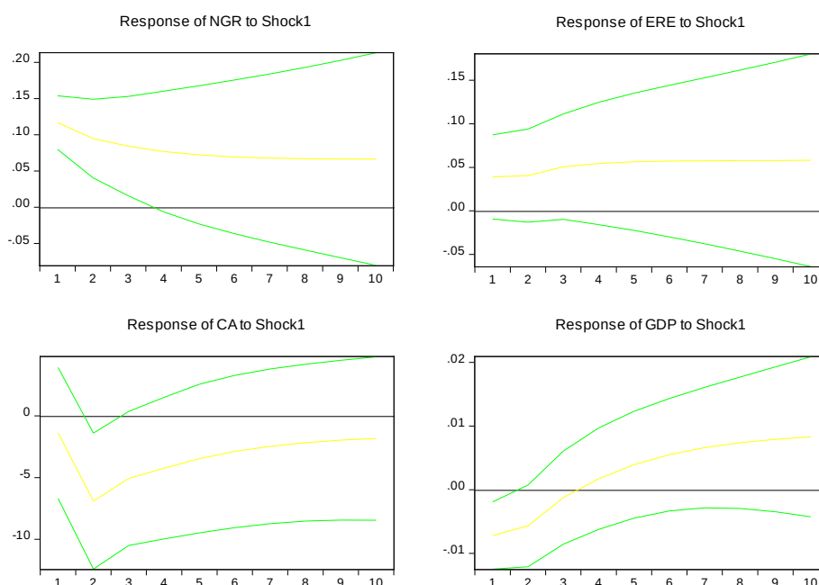
شکل ۱: نمودار ضربه- واکنش متغیرها به شوک قیمت گاز طبیعی
